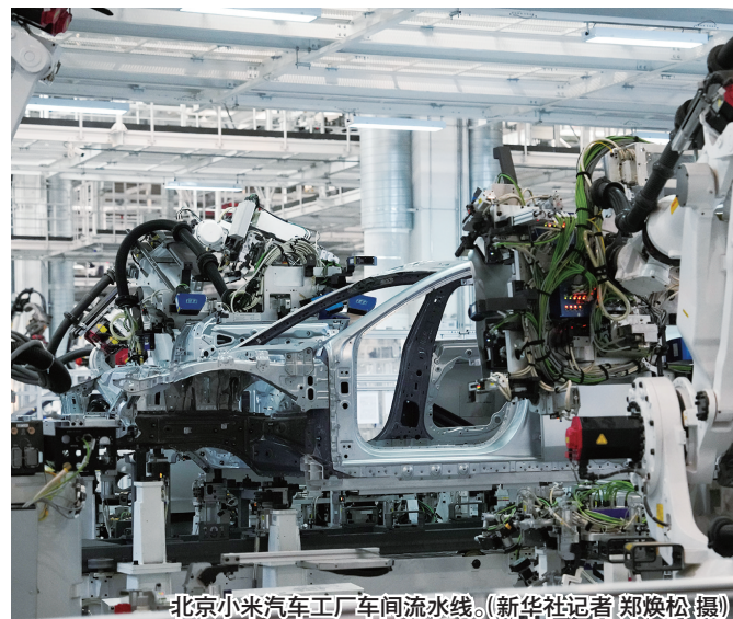
北京小米汽车工厂车间流水线。(新华社记者 郑焕松摄)
