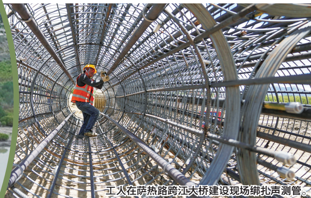
工人在萨热路跨江大桥建设现场绑扎声测管。
