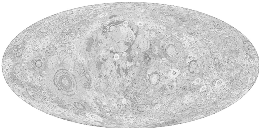
月球地质图
