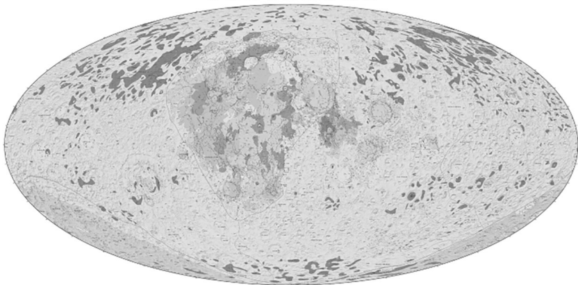
月球岩石类型分布图
