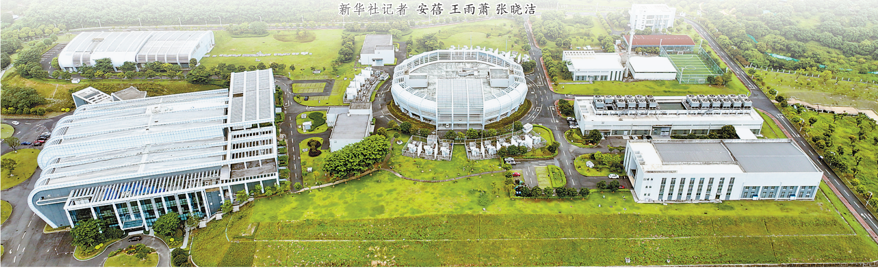
在粤港澳大湾区多地,一系列在建和已启用的大科学装置集群效应初现,助力大湾区加速迈向国际科技创新中心。图为在广东东莞拍摄的中国散裂中子源(2024年7月8日摄,无人机照片)。
