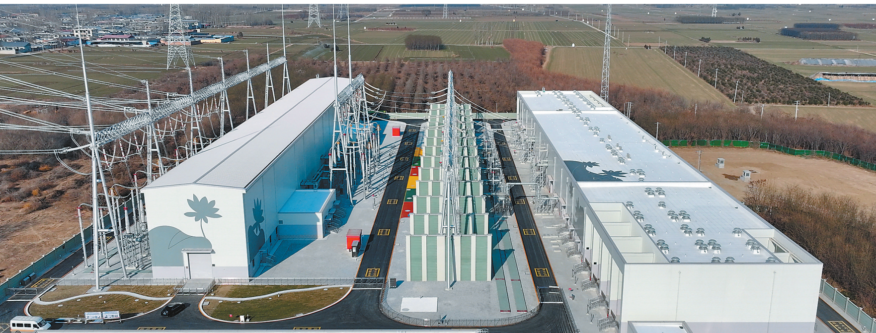
12月7日，雄安新区新能源输送通道关键枢纽变电站——雄安500千伏超高压变电站正式投运。据介绍，该变电站是国家“十四五”规划重点项目，是将内蒙古和河北坝上地区风电、光伏发电等清洁能源引入雄安新区的关键站点。 图为12月6日拍摄的雄安500千伏超高压变电站(无人机照片)。
