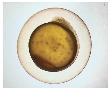
胚胎发育图。
