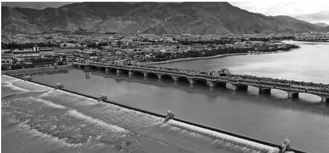
拉萨河综合整治工程5#闸。图由拉萨市水利局提供
